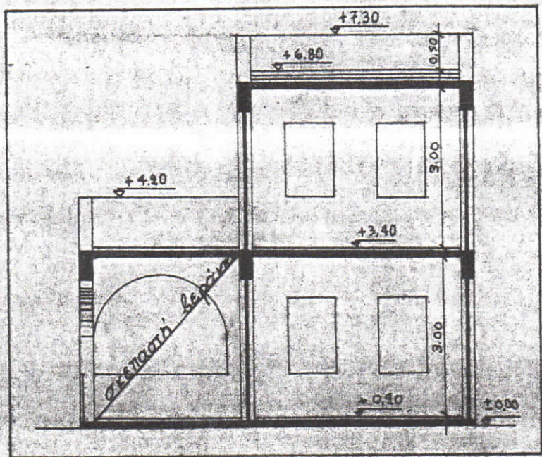
ΣΧΗΜΑΤΙΚΗ ΤΟΜΗ 1-1'
